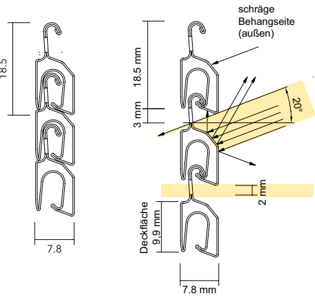
Profile geschlossen (Ansicht von außen)
