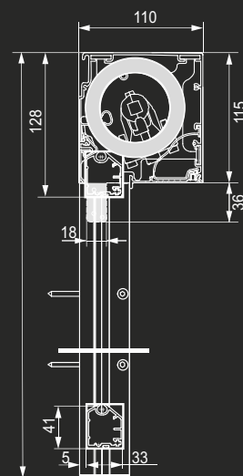
Querschnitt Führungsschiene Maßangaben in mm
